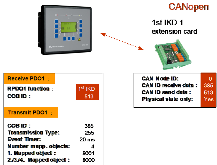
Figure 4-4: CANopen Schnittstelle - Einstellungen für externe Geräte
