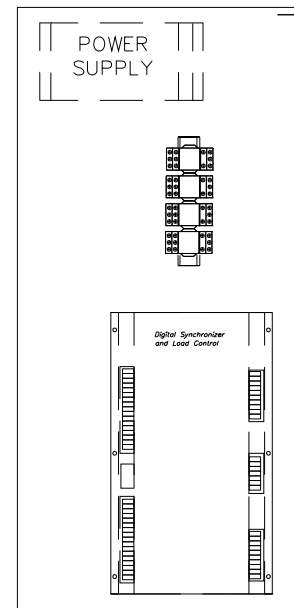
OPTIONAL DSCL PANEL
