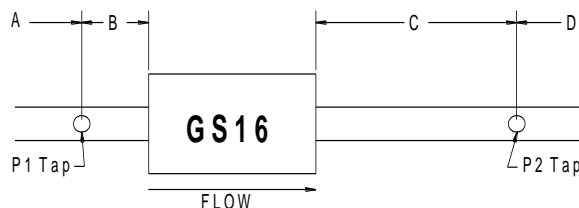
图 2-1. 管道要求
