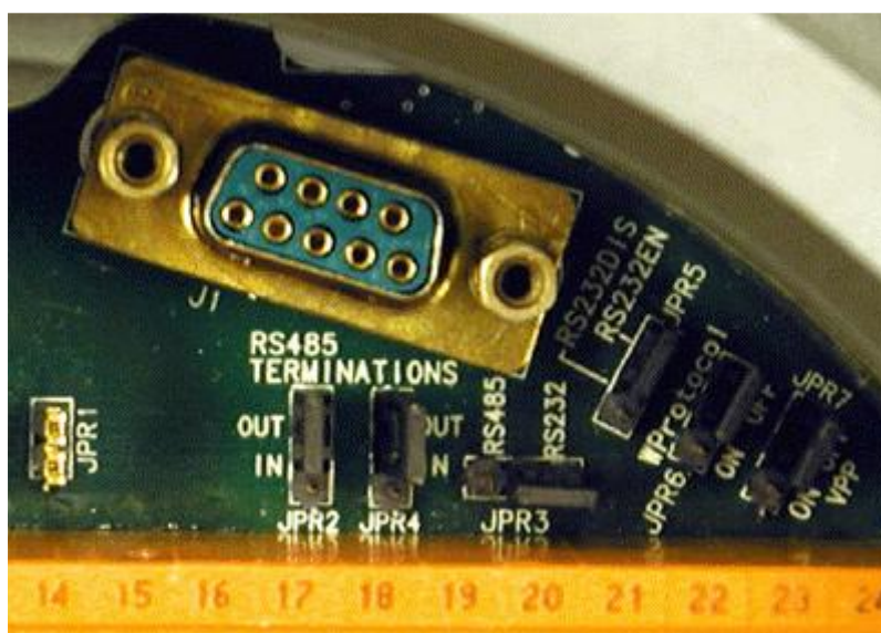
图 2-7b. 服务端口(特写)
