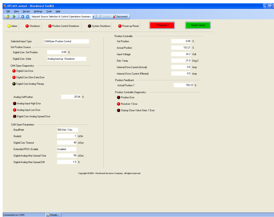
图 4-18. CANopen 位置控制
