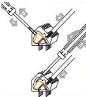
图 2-2. WAGO 接线端子
