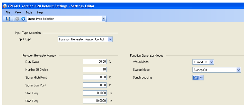
图 4-32. 函数发生器位置控制
