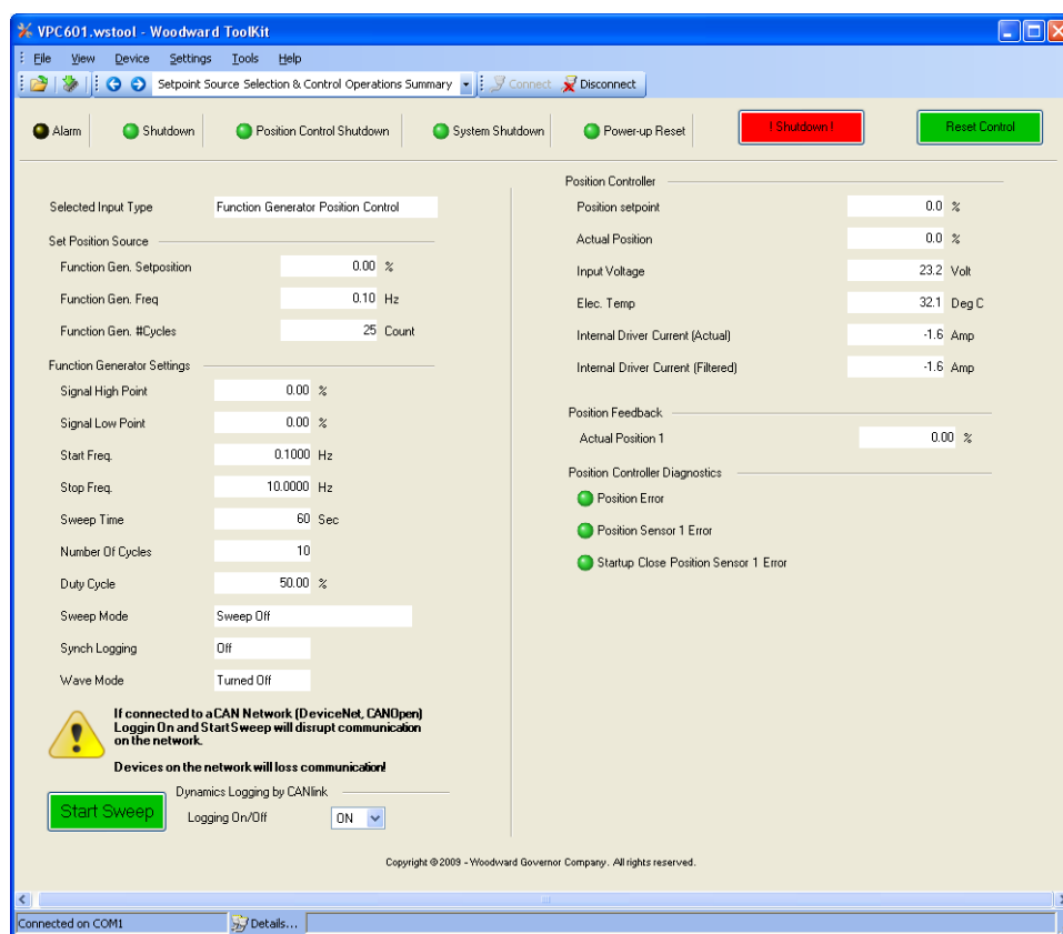
图 4-19. 函数发生器位置控制
