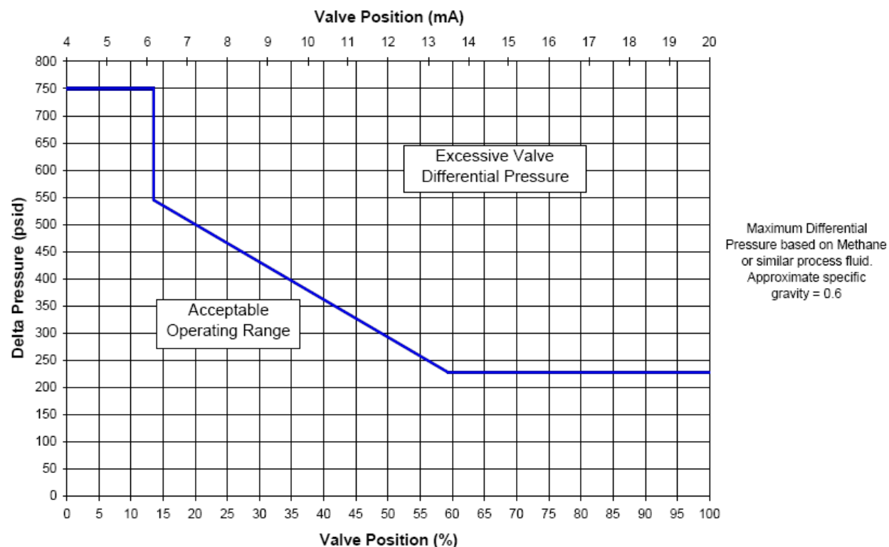
图 3-3. GS16 1.5 端口最大阀门差压
