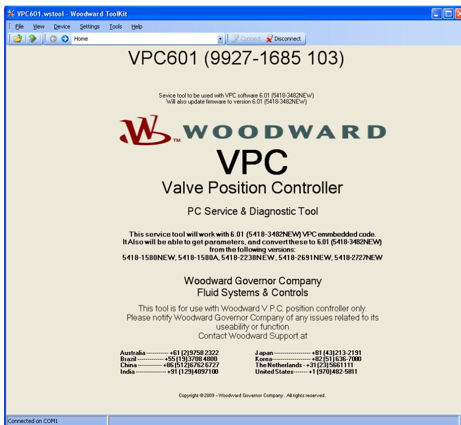
图 4-1. VPC 标题页面
