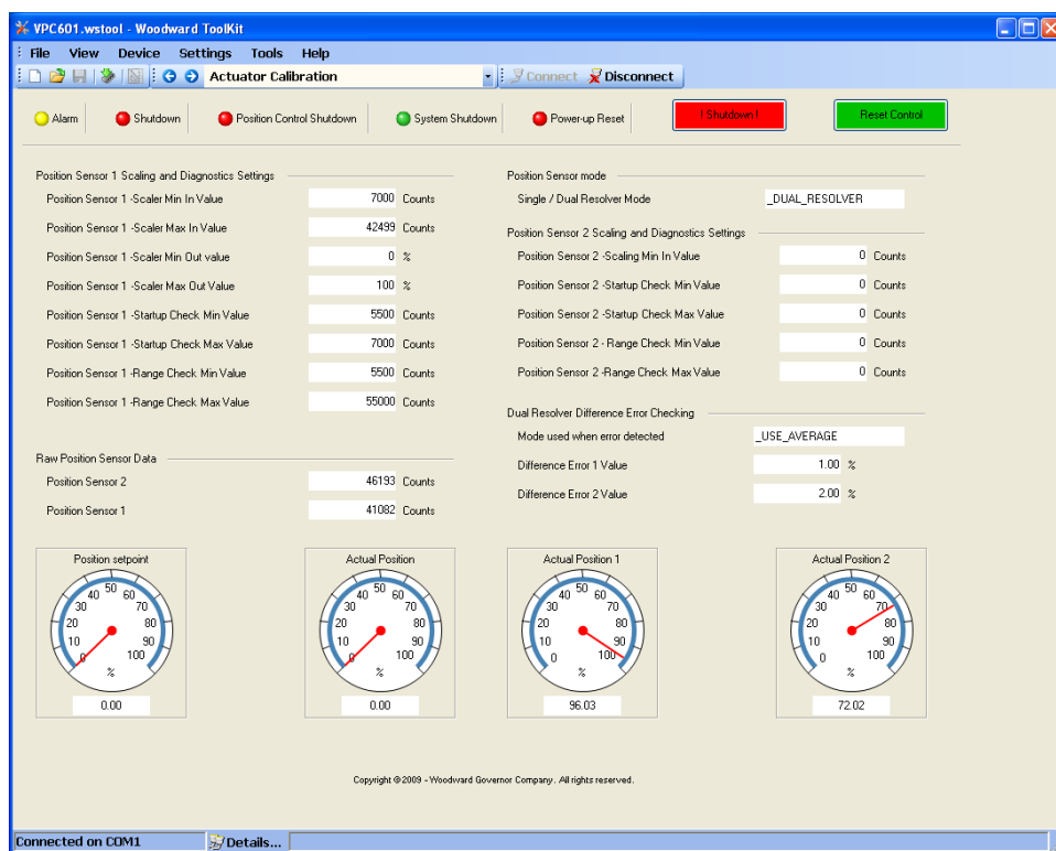
图 4-21. 双变压器执行器
