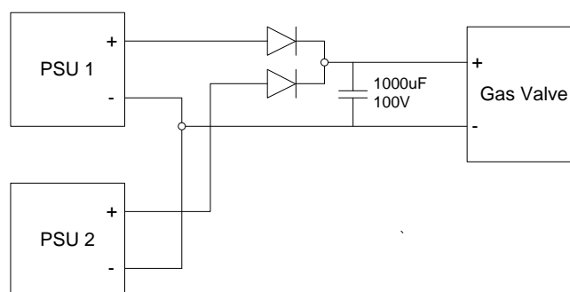
图 2-5. 推荐的并联电源连接
