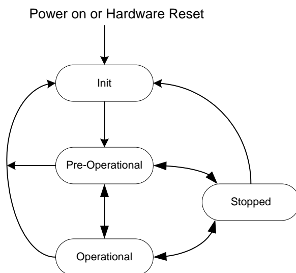
图 3-1. CANopen 状态图
