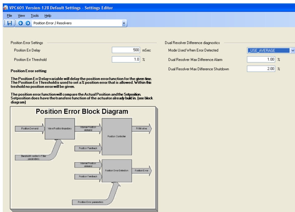
图 4-35. 位置错误/旋转变压器设定页面
