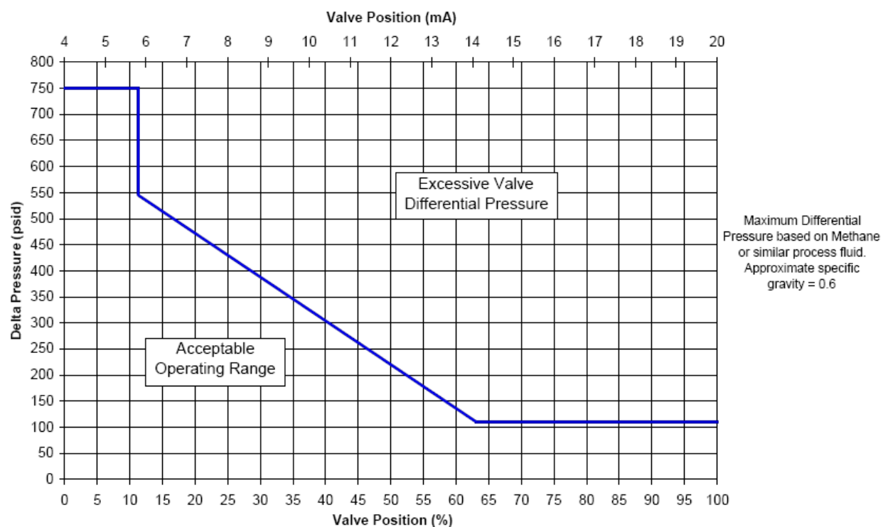
图 3-4. GS16 2.0 端口最大阀门差压
