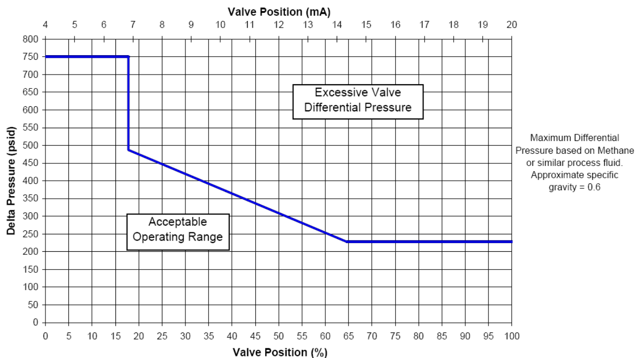
图 3-2. GS16 1.0 端口最大阀门差压
