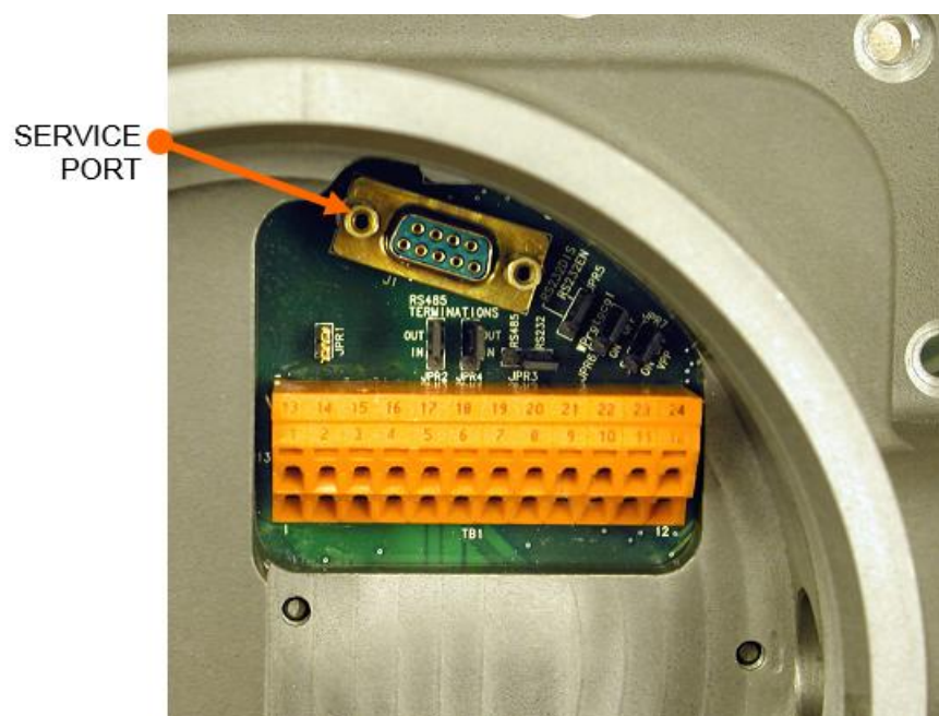
图 2-7a. 服务端口
