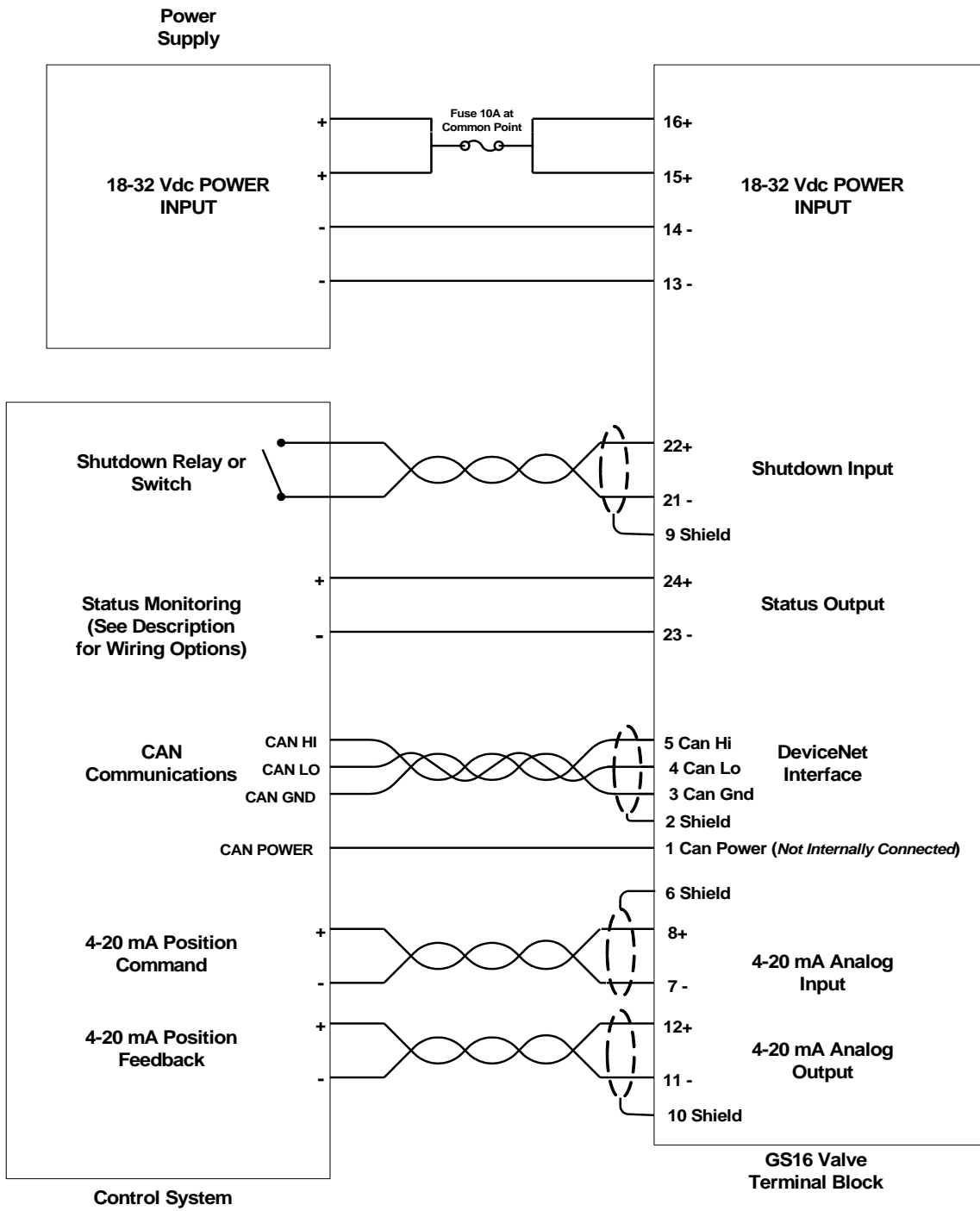
图 2-4. GS16 工厂接线图
