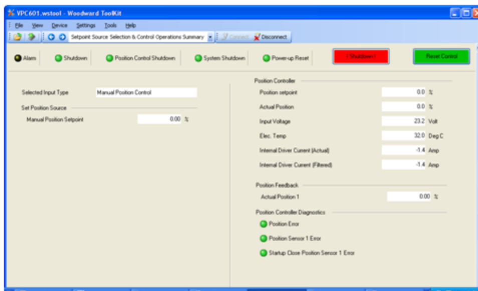
图 4-17. 手动位置控制
