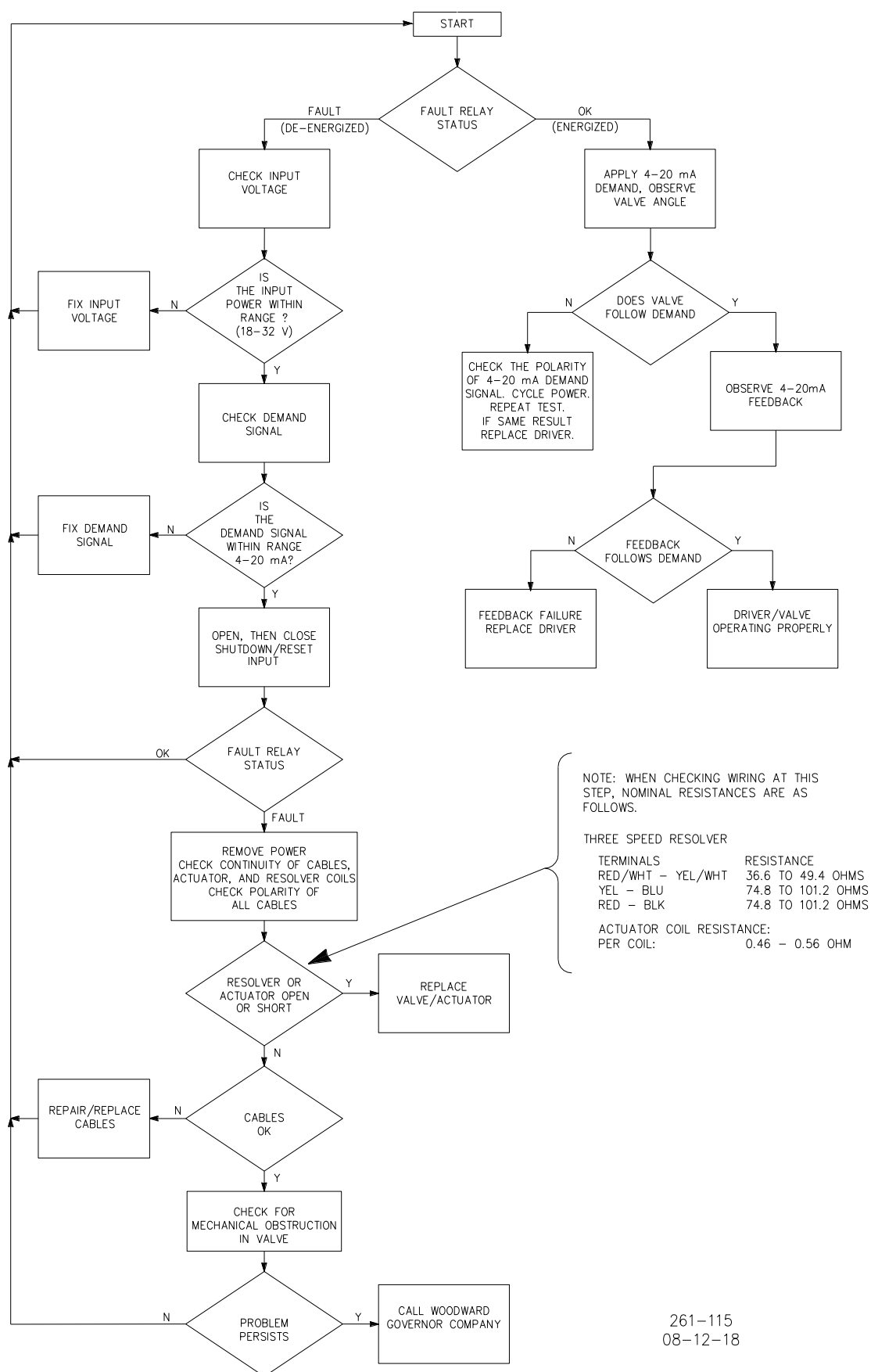
图 7-1. 故障排除流程图
