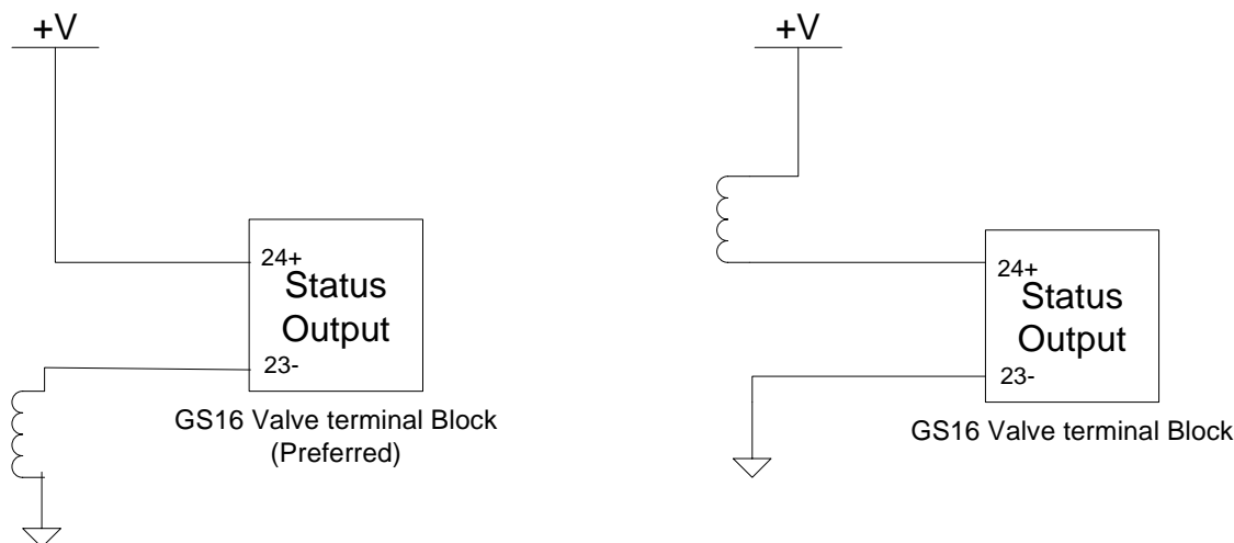
图 2-6. 状态输出接线示例
