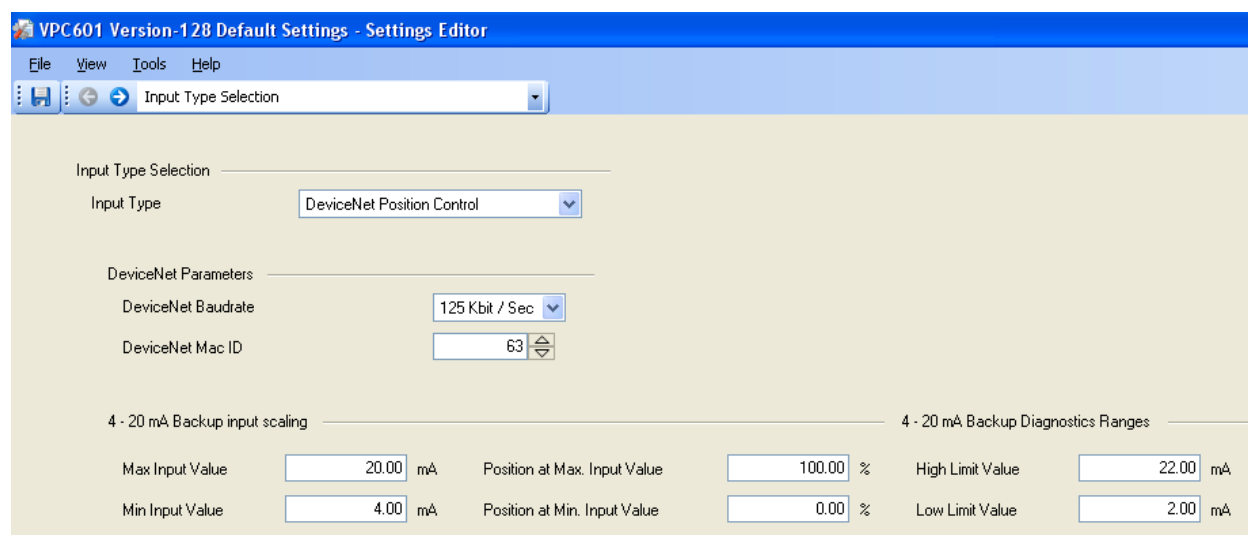
图 4-31. DeviceNet 位置控制
