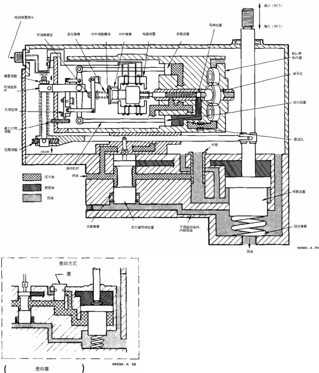
5.25-英寸液力放大器原理图
