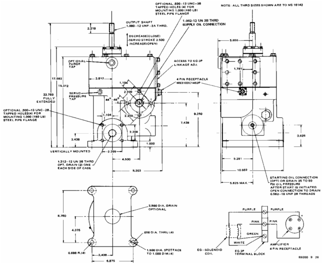
典型的5.25-英寸液力放大器外形图（尺寸仅供参考）
