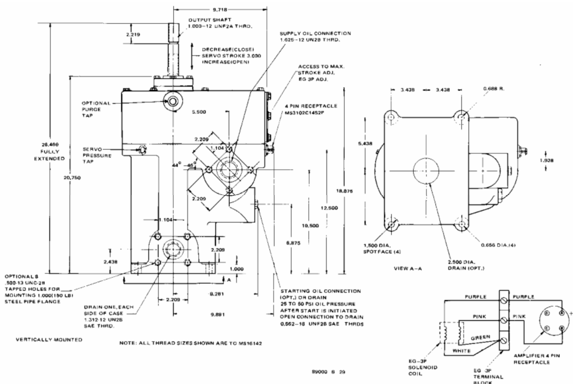
典型的7.25-英寸液力放大器外形图（尺寸仅供参考）
