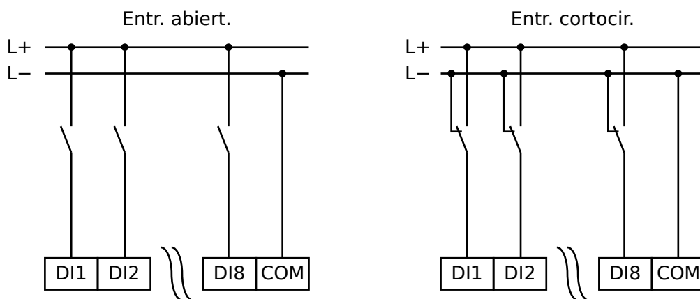
Fig. 80: Estado seguro de entradas digitales
