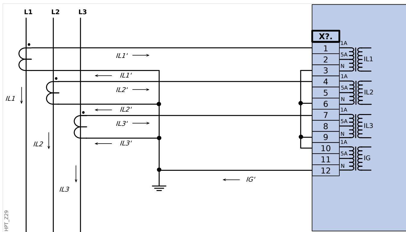
Fig. 22: Medida corriente trifásica; En secundario = 1 A. Medic corr de tierra mediante conexión Holmgreen; IGnom secund = 1 A.
