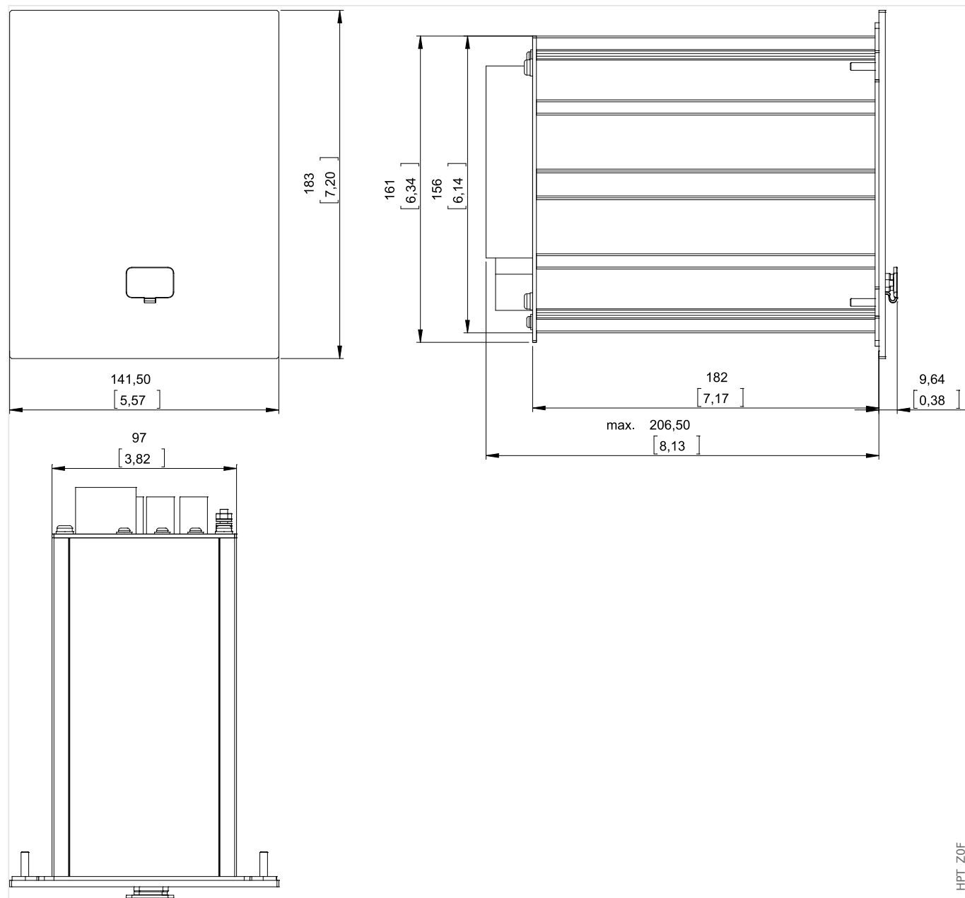
Fig. 5: Vista de 3 lados, carcasa B1 (dispositivos con 8 teclas) Todas las dimensiones se expresan en mm, excepto las dimensiones entre paréntesis [pulg.]
