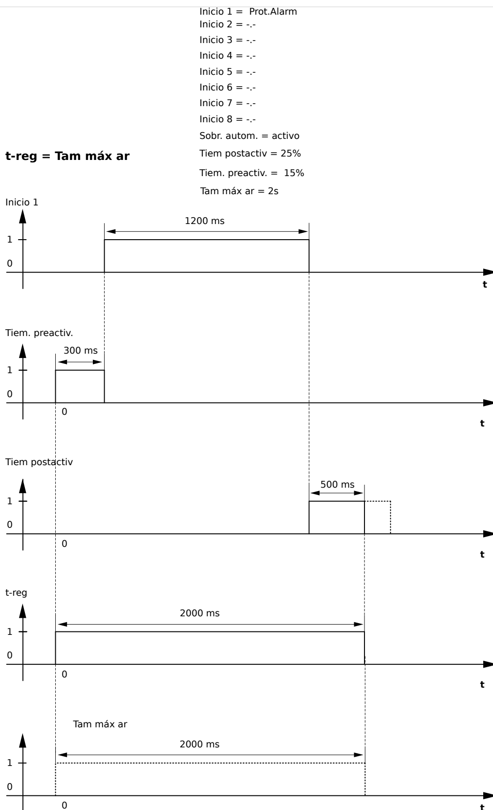
Fig. 69: Ejemplo 1: cuadro de intervalos del registrador de perturbaciones
