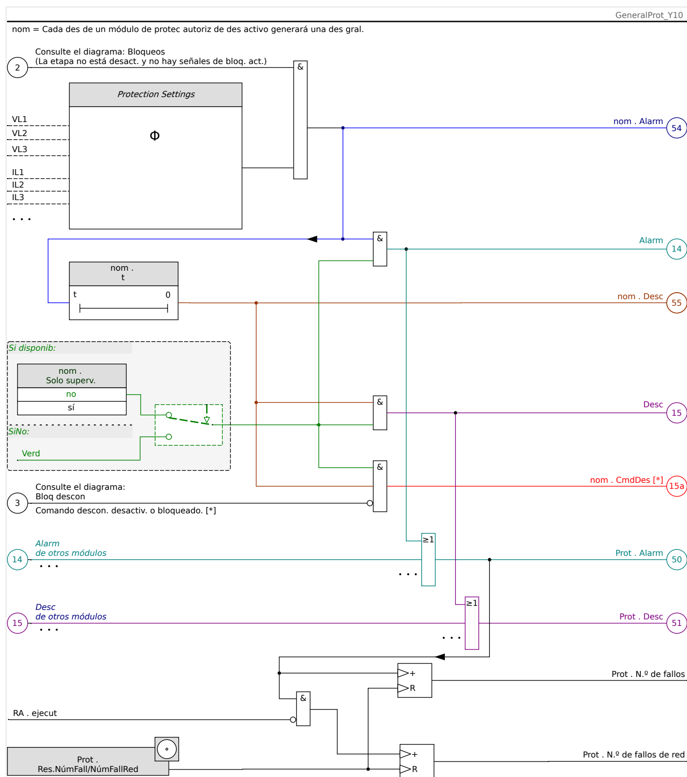
Fig. 43: Descripción a grandes rasgos de la funcionalidad de cualquier elemento de protección de HighPROTEC.
