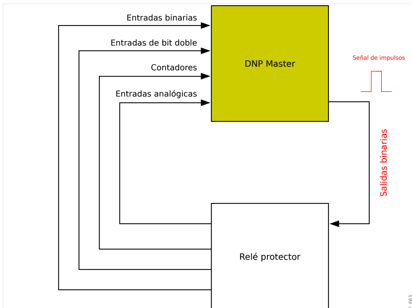
Fig. 39: Asignación de puntos
