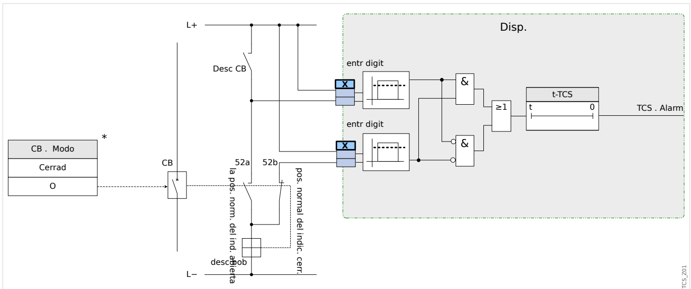
Fig. 58: Ejemplo de conexión: Supervisión del circuito de desconexión con dos contactos auxiliares CB »Aux ON« (52a) and »Aux OFF« (52b).
