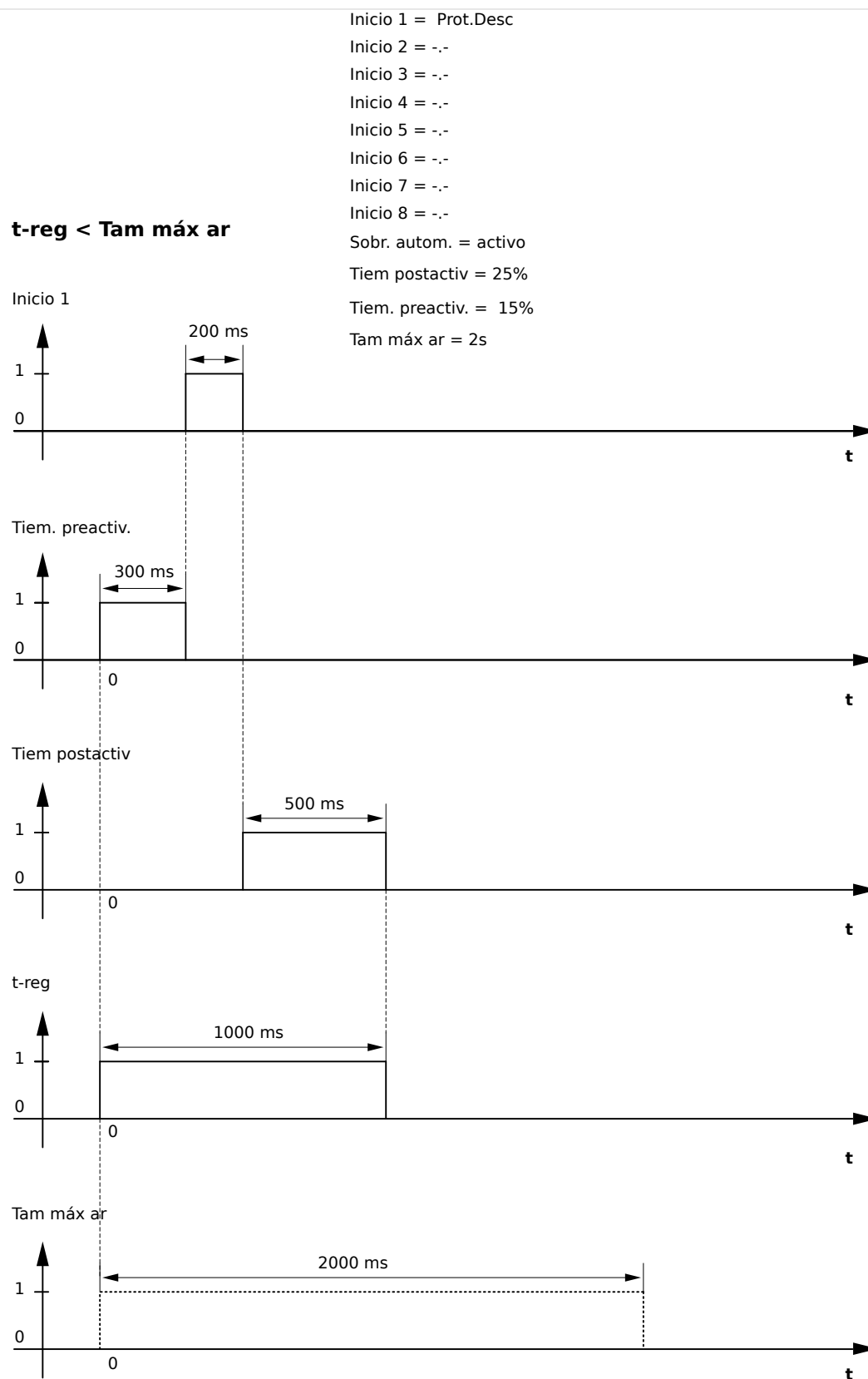
Fig. 70: Ejemplo 2: cuadro de intervalos del registrador de perturbaciones
