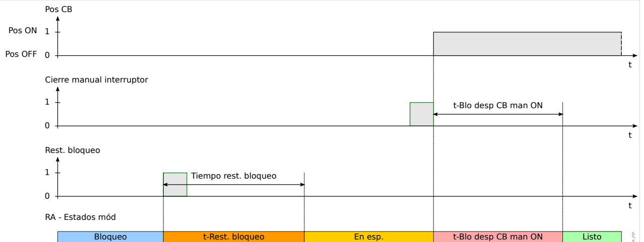
Fig. 54: Lógica de reinicio de bloqueo de AR en caso de que el reinicio de bloqueo llegue antes de que se cierre el interruptor manualmente.
