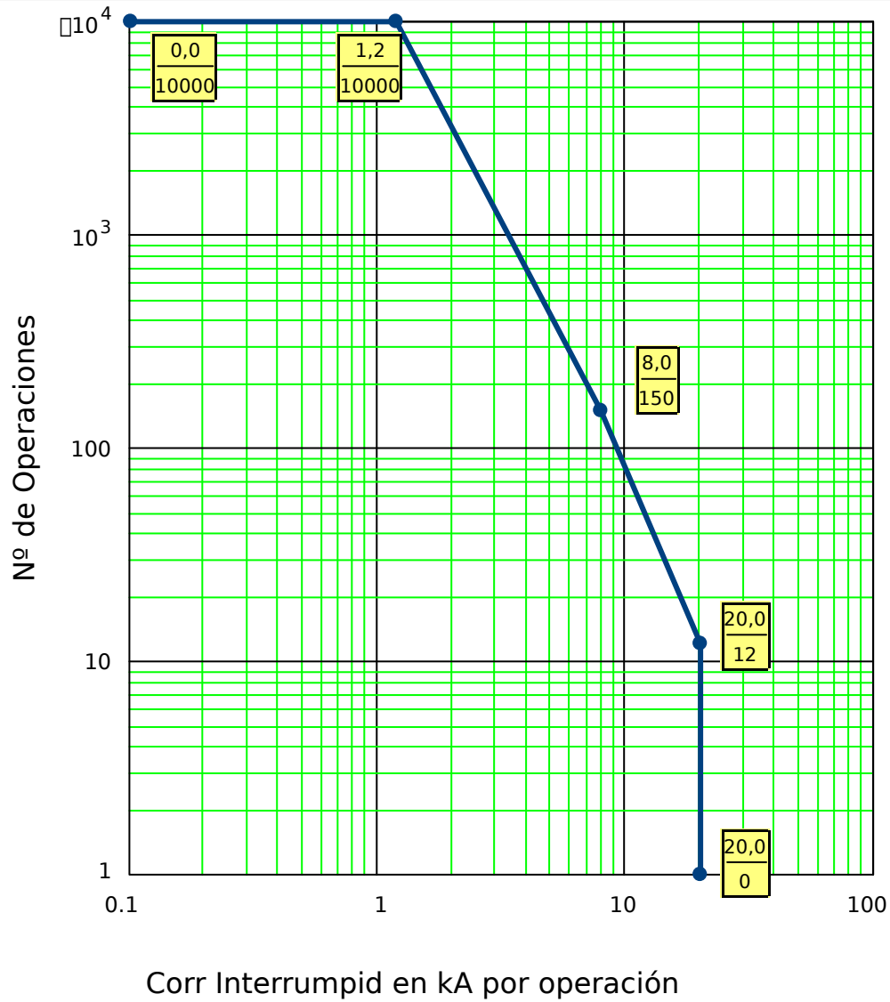
Fig. 66: Curva Mantenim Interruptor para Interrupt Circuito típico 25kV
