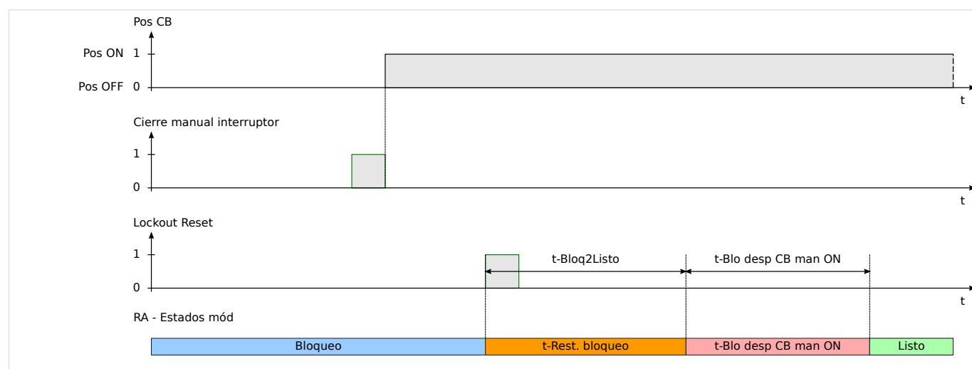
Fig. 55: Lógica de reinicio de bloqueo de AR en caso de que el reinicio de bloqueo llegue después de que se cierra el interruptor manualmente.
