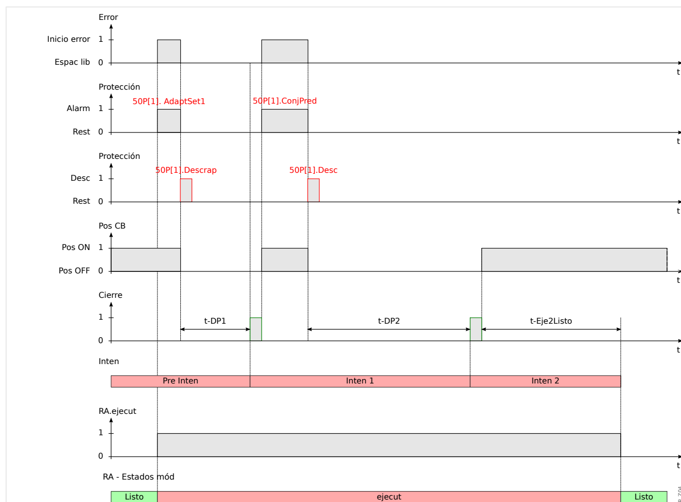
Fig. 51: Diagrama de tiempo de reconexión automática para el esquema de reconexión automática de dos intentos successful (correctos) con aceleración en un intento previo.
