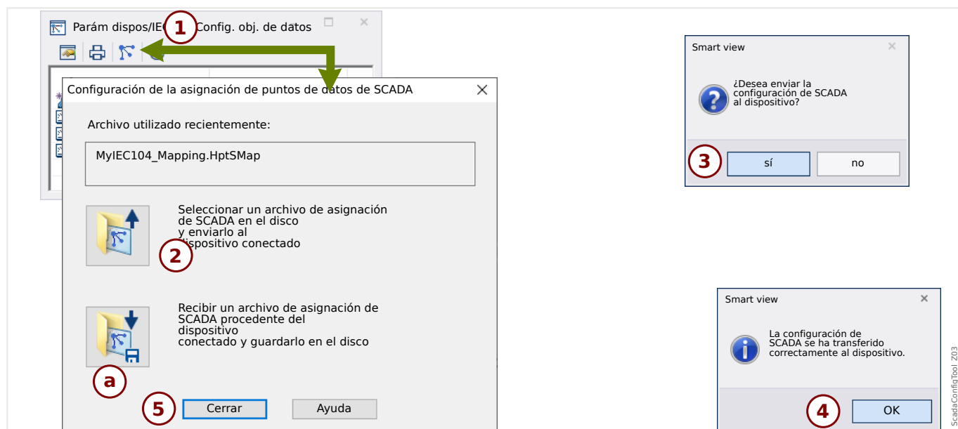
Fig. 41: Ejemplo de uso de Smart view para transferir el archivo *.HptSMap al dispositivo de protección.
