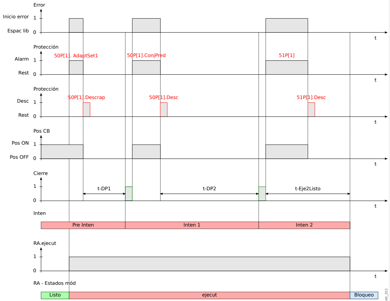
Fig. 50: Diagrama de tiempo de reconexión automática para el esquema de reconexión automática de dos intentos unsuccessful (incorrectos) con aceleración en un intento previo.
