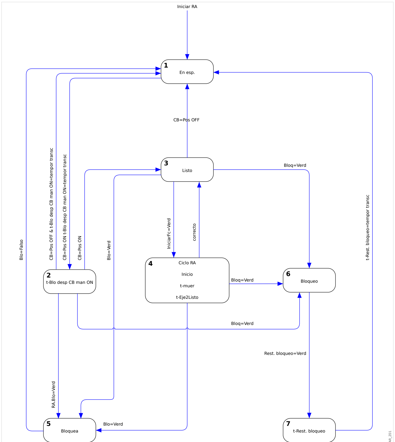
Fig. 48: Diagrama de transición de estado.
