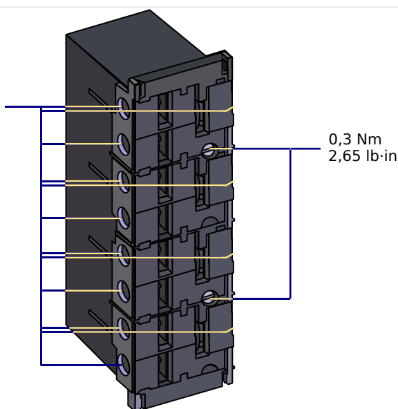
Fig. 79: Conector enchufable con cortocircuitador integrado (entradas de corriente convencionales)
